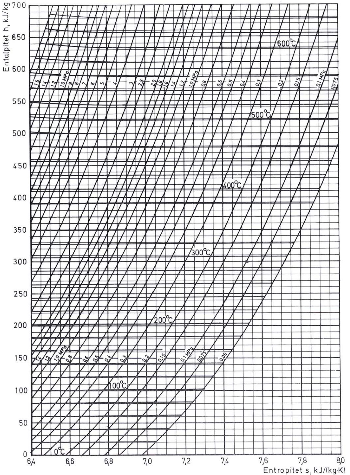
sh-diagram för torr luft
