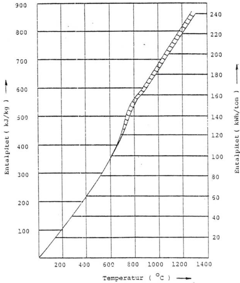
Specifika entalpin vid olika temperaturer. Sammanställt utifrån mätdata för olika kolstål.
