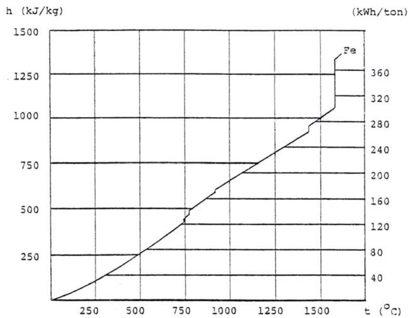
Diagram som beskriver järns entalpi som funktion av temperaturen
