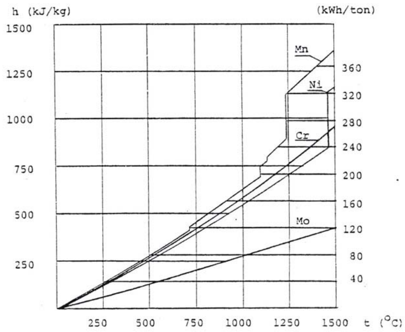
Olika legeringsämnenens entalpi som funktion av temperaturen.
